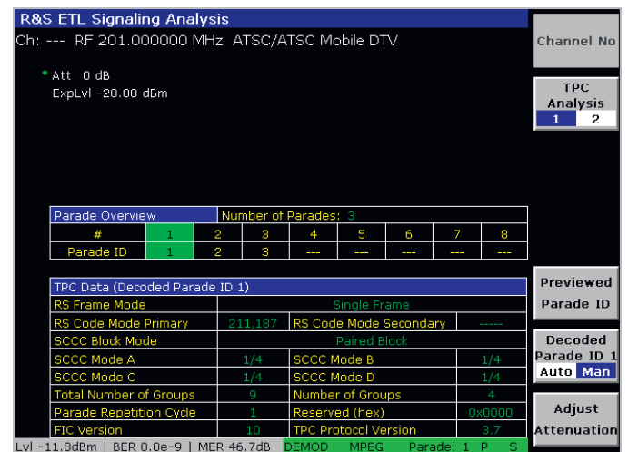
Anzeige der dynamischen Belegung von ATSC-M/H Subframes
